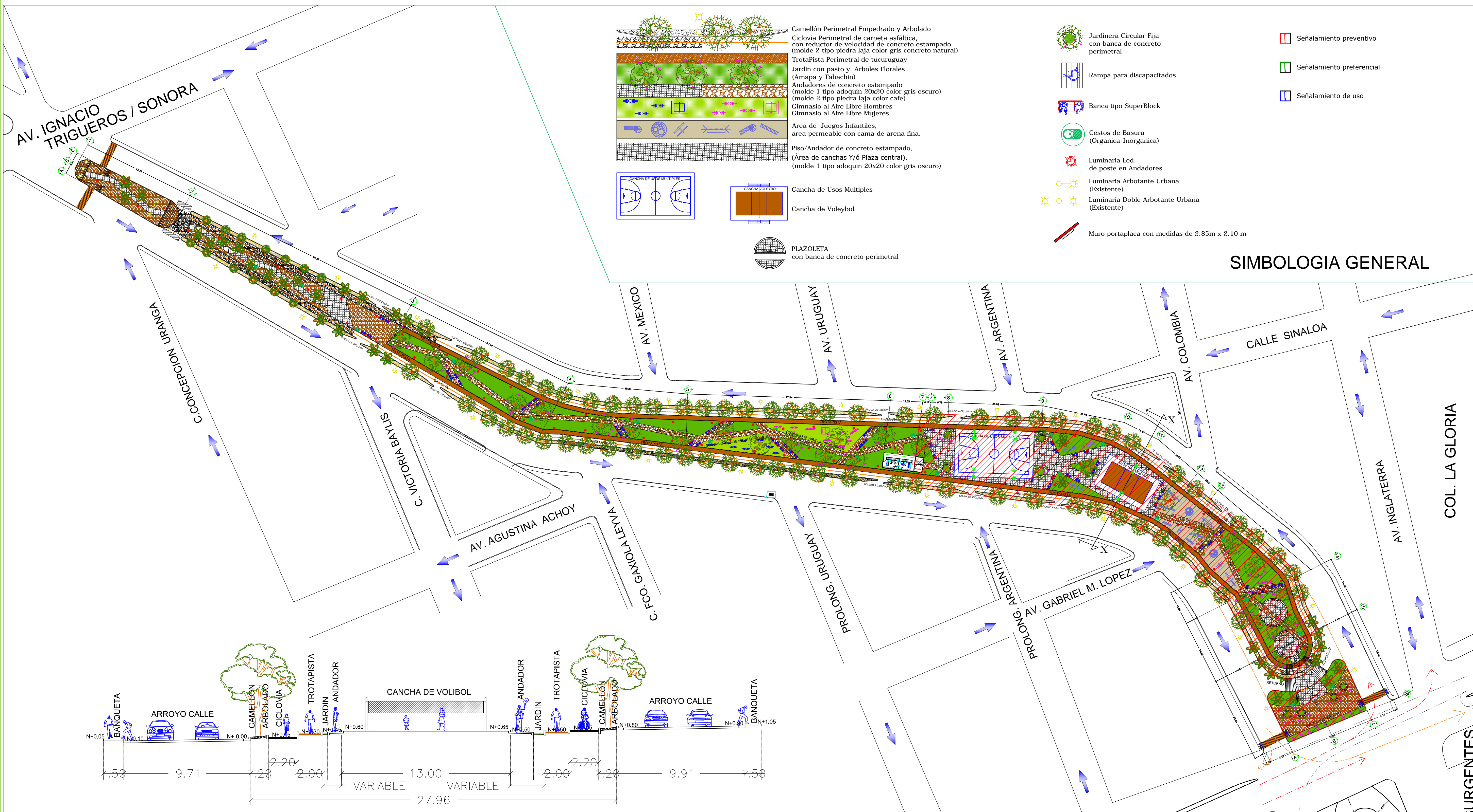
CORTE-ALZADO TRANSVERSAL X-X' SIN ESCALA
