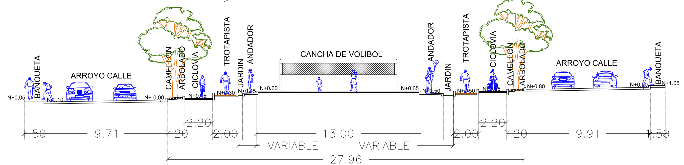
CORTE-ALZADO TRANSVERSAL X-X' SIN ESCALA
